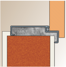
AGAT Montaż bez dodatkowych elementów kotwiących.
