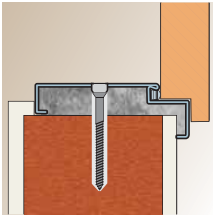
OPAL Montaż na dyble.
