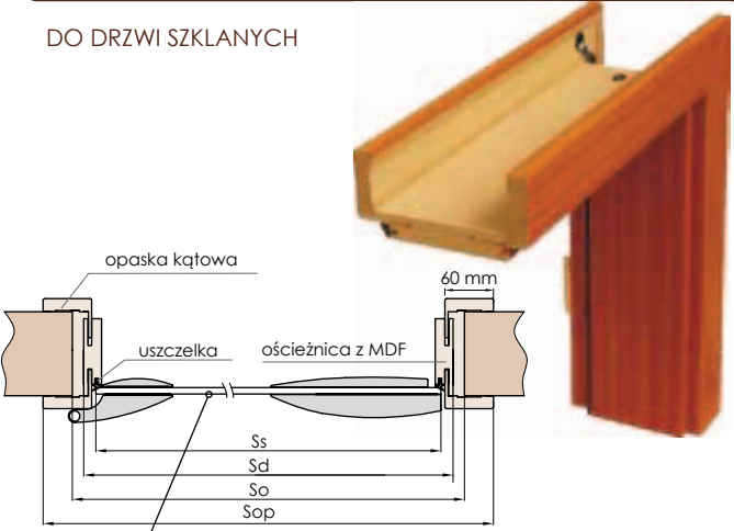
01 TAFLA SZKLANA I satyna 02 01 TAFLA SZKLANA II 02
