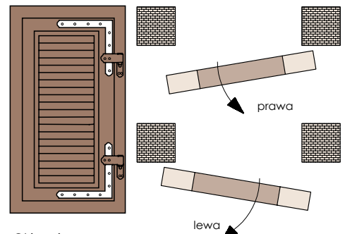
Okiennica dwuskrzydłowa
