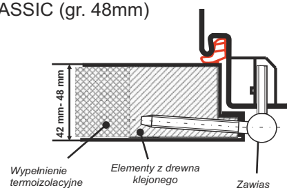
PRZEKRÓJ SKRZYDŁA - EKO, STANDARD, (gr. 42mm) CLASSIC (gr. 48mm)
