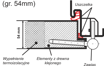
PRZEKRÓJ SKRZYDŁA - PLUS I STANDARD 55 (gr. 54mm)
