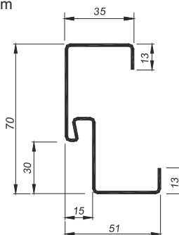
OŚCIEŻNICA KMT EKO
